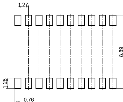
P.C.B. LAYOUT
